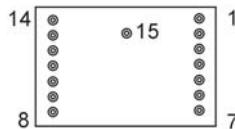
Рис.1 Расположение выводов (вид снизу).
