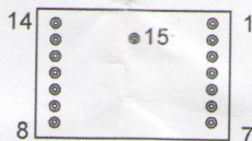
Рис.1 Расположение выводов (вид снизу).
