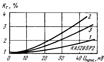
Типовые зависимости коэффициента гармоник БИС КА528БР2 от напряжения пульсаций источника питания и генератора тактовых импульсов:
