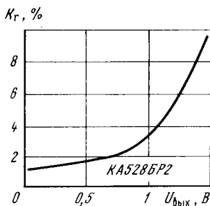
Типовая зависимость коэффициента гармоник БИС КА528БР2 от выходного напряжения
