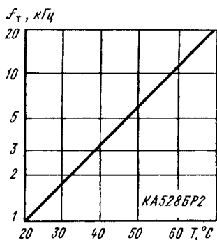
Типовая зависимость частоты управляющих тактовых импульсов КА528БР2 от температуры окружающей среды
