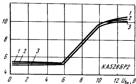
Типовые передаточные характеристики БИС KA528BP2:
