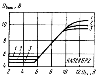
Типовые передаточные характеристики БИС КА528БР2:
