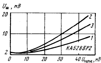
Типовые зависимости напряжения шумов, приведенных ко входу БИС КА528БР2, от напряжения пульсаций источника питания и генератора тактовых импульсов:
