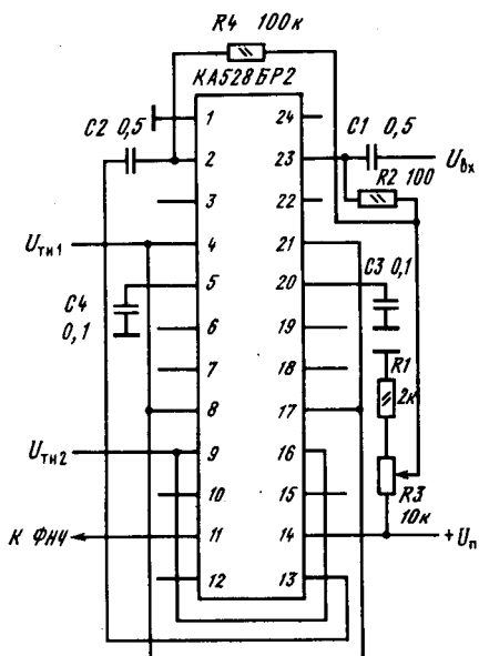
Типовая схема включения БИС КА528BP2
