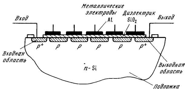
Структура ПЗС типа «пожарная цепочка»
