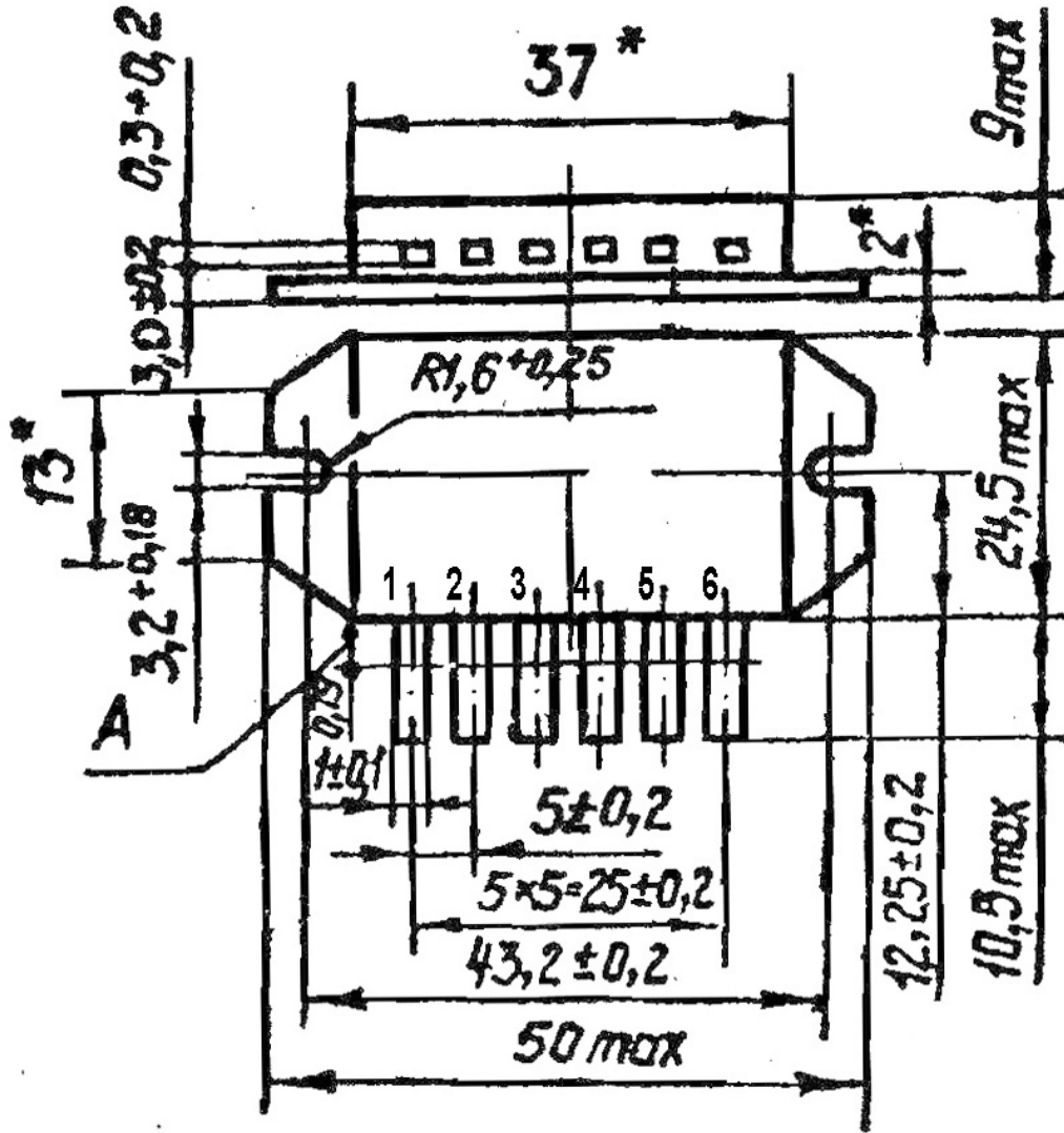
Габаритный чертеж корпуса
