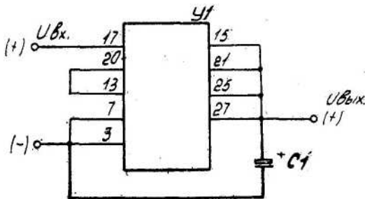
У1 - стабилизатор; С1 - конденсатор 50 мкФ +80-20% Рис. 5.3
