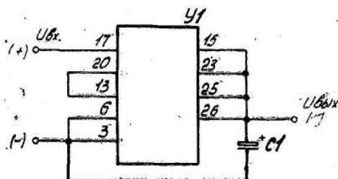
У1 - стабилизатор; С1 - конденсатор 50 мкФ +80-20% Рис. 5.2
