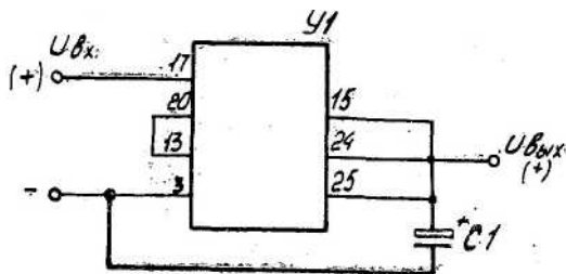
У1 - стабилизатор; С1 - конденсатор 50 мкФ +80-20% Рис. 5.1
