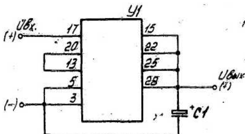
У1 - стабилизатор; С1 - конденсатор 50 мкФ +80-20% Рис. 5.4
