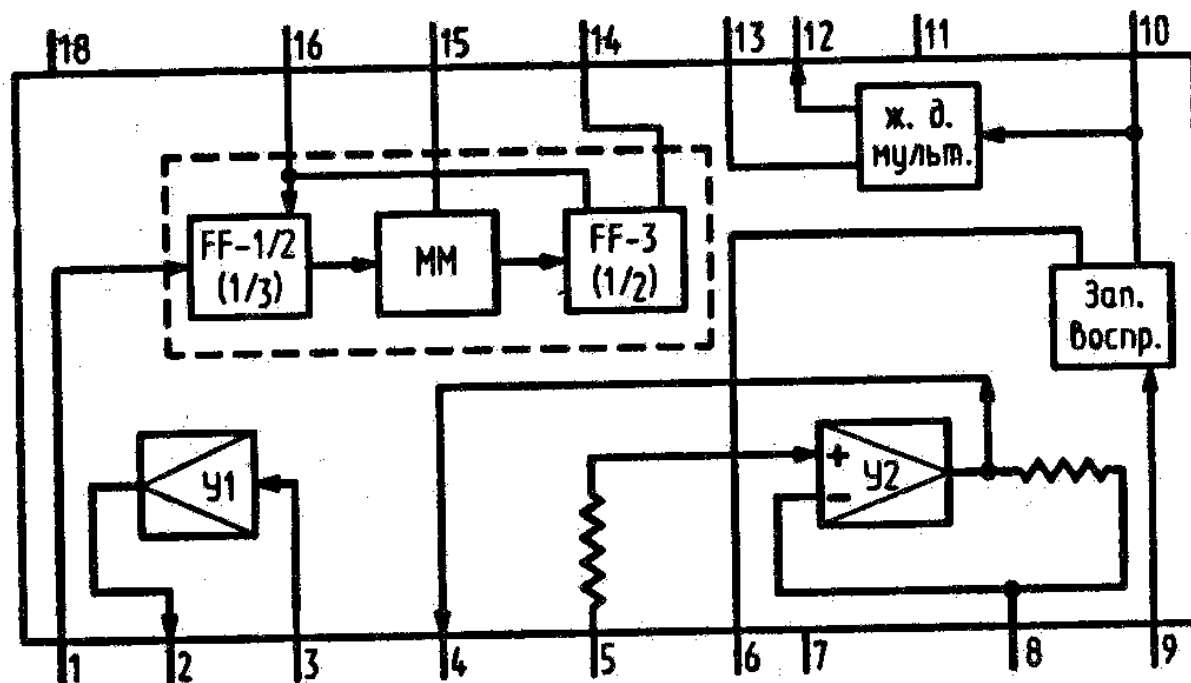
Функциональная схема
