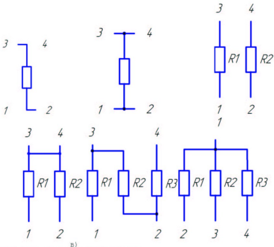
Рисунок 1 Мощные резисторы разработки НИИЭМП:
